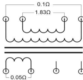
Tr1, F-TXFORMER---117
